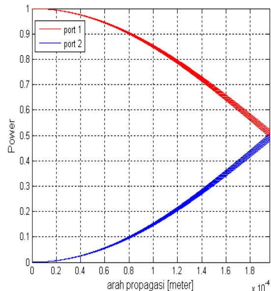
Gambar 8. Daya keluaran kedua pandu gelombang sebesar 3\text{ dB}
