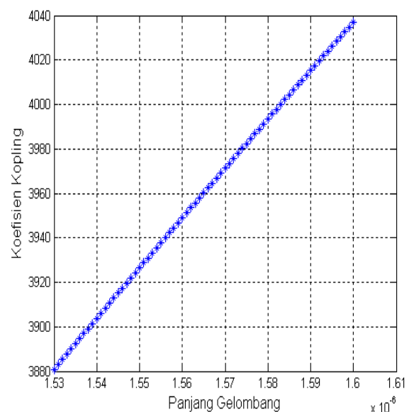
Gambar 5. Hubungan koefisien kopling dan panjang gelombang
