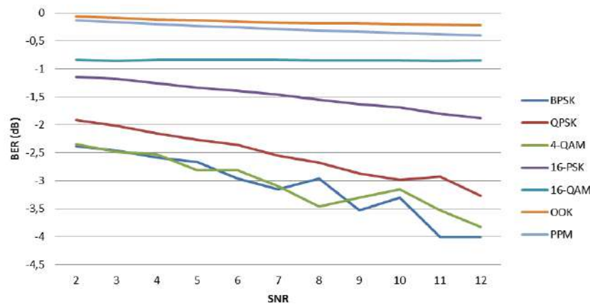
Gambar 3. BER Berbagai Modulasi untuk SNR 2-12 pada Iradiasi 0,7
