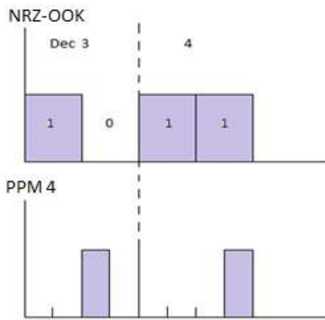
Gambar 2. OOK 2 Bit dan PPM 4 Slot Waktu.
