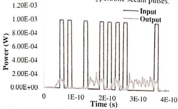
Fig. 4 Input and output of Fiber non-soliton parameter (using RZ pulse)
