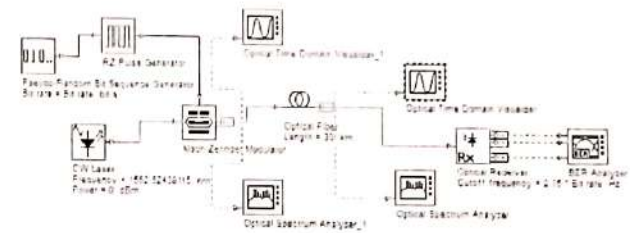
Fig. 2 Design Fiber non-soliton parameters [1].
