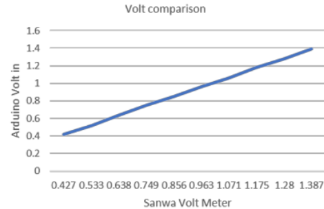
Fig. 11. Volt comparison
